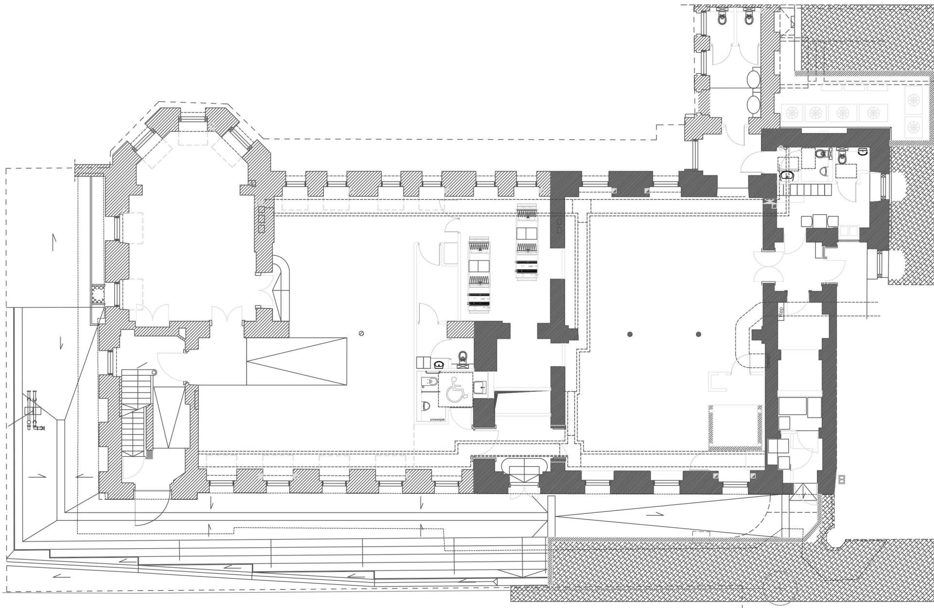
KONDYGNACJA 1
